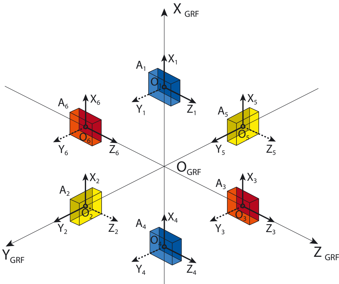
Abb. 3: Gradiometerprinzip. Die paarweisen Differenzen zwischen den Beschleunigungsmessern liefern die Schweregradienten.
