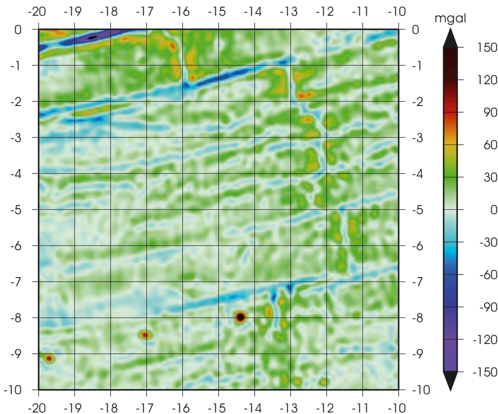
Abb. 5: Schwereanomalien aus einem regionalen Schwerefeldmodell des DGFI, basierend auf Daten der Altimetermissionen ERS-1 und CryoSat sowie GOCE-Messungen.
