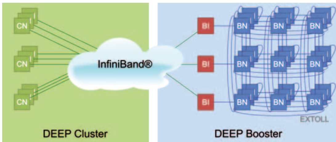
Cluster-Booster-Architektur des DEEP-Prototypen.
